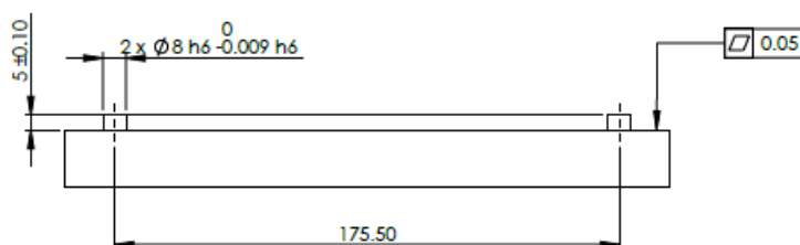
1.2: Szerelőlemez robotalaphoz
